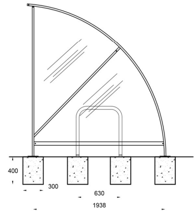
END ELEVATION
