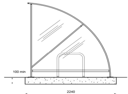
END ELEVATION
